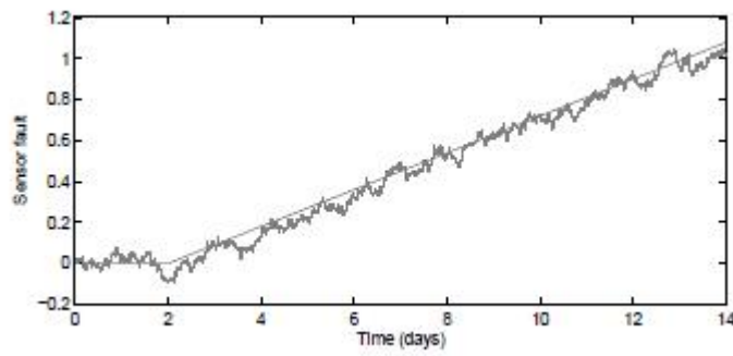
FIGURE 4.6 – Défaut dérive
