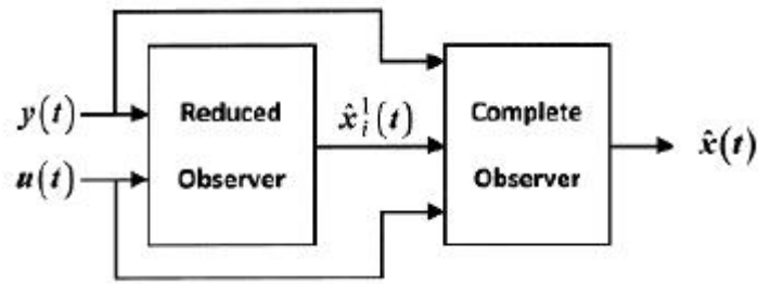
FIGURE 4.1 – Observateur en cascade
