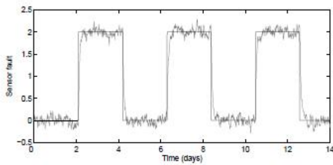
FIGURE 4.7 – Défaut intermittent
