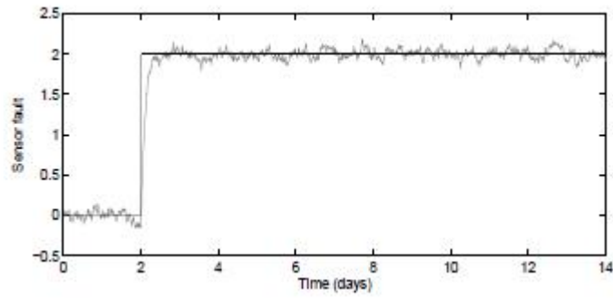
FIGURE 4.5 – Défaut échelon
